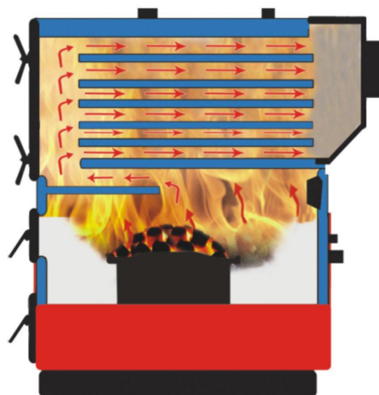
трехходовой теплообменник
