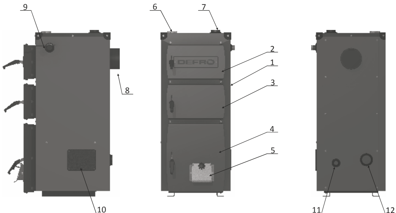
Рисунок 4. Основные элементы котла.
