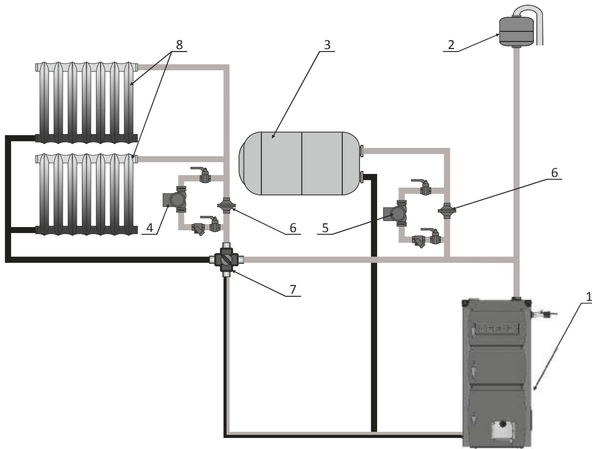
Рис. 11. Схема общего подключения перекрестного клапана к отопительной системе 1 - котел, 2 - расширительный бак открытого (закрытого) типа, 3 - бак горячей воды 4 - насос ц.о, 5 - насос г.в.с, 6 - дифференциальный клапан, 7 - перекрестный клапан, 8 - батареи
