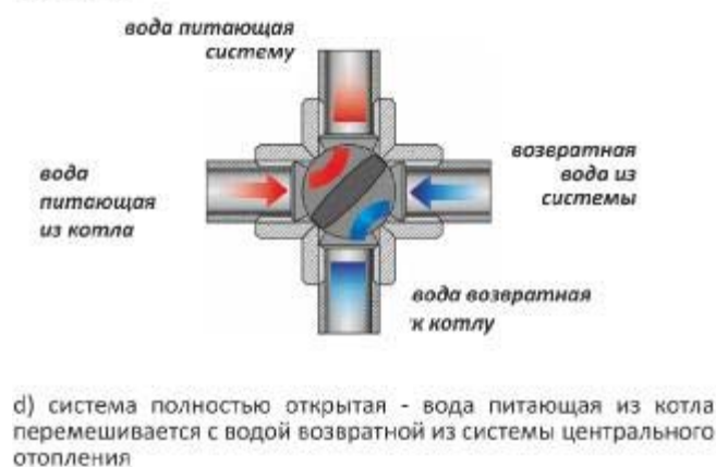
Рис.10 а)-д) Схема работы перекрестного клапана
